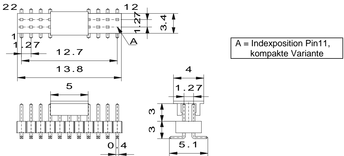
Bild 4: Stecker-Leiste für Systemplatine
