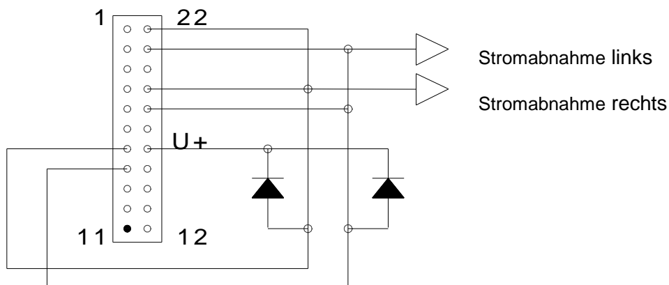
Bild 7: Typischer Brückenstecker
