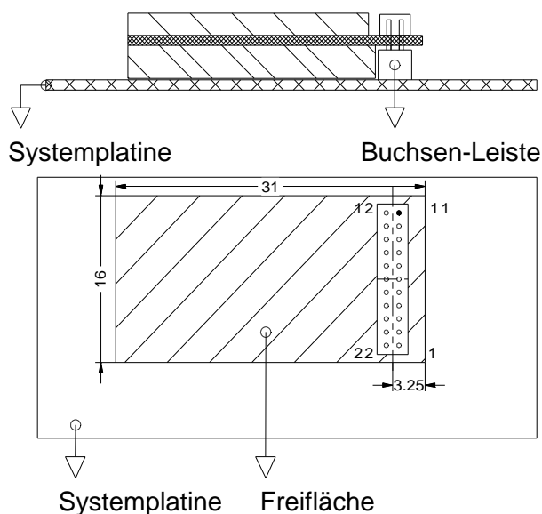
Bild 5: Kompakte Variante
